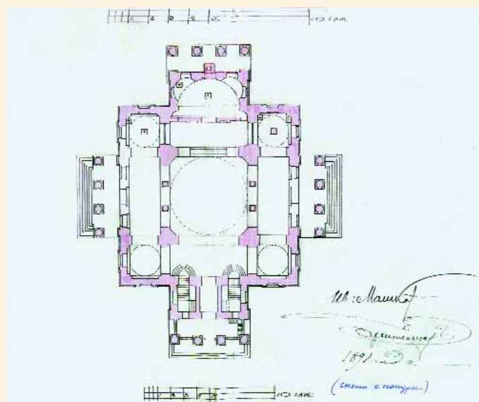
План Троицкого храма. Рисунок И.П. Машкова. 1891 г. ЛОКМ
